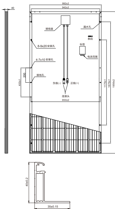
产品图示 单位: mm
